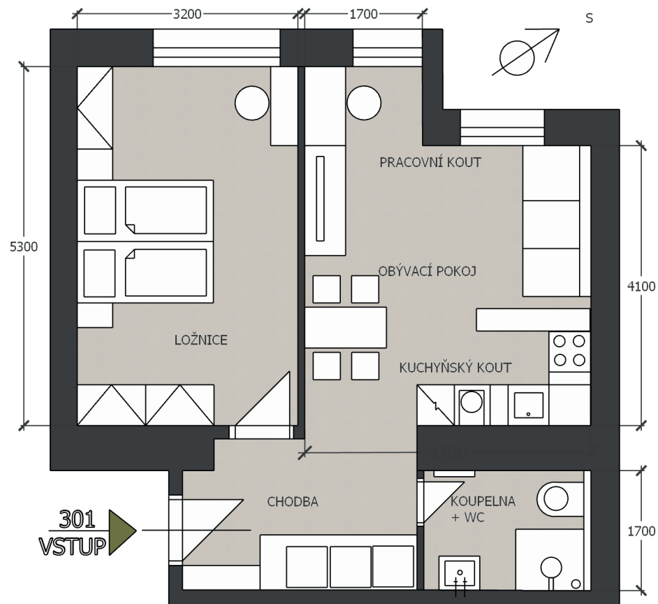
PŮDORYS
